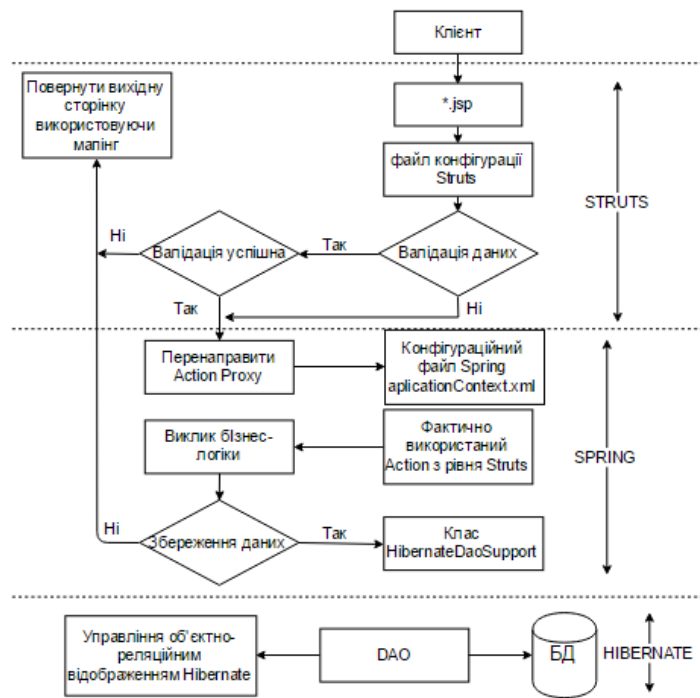
Рис. 3 – Принцип взаємодії Hibernate, Struts, Spring
