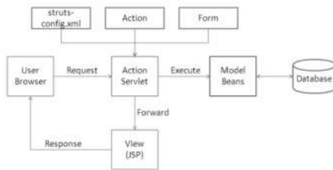
Рис. 2 – Типова архітектура Struts
