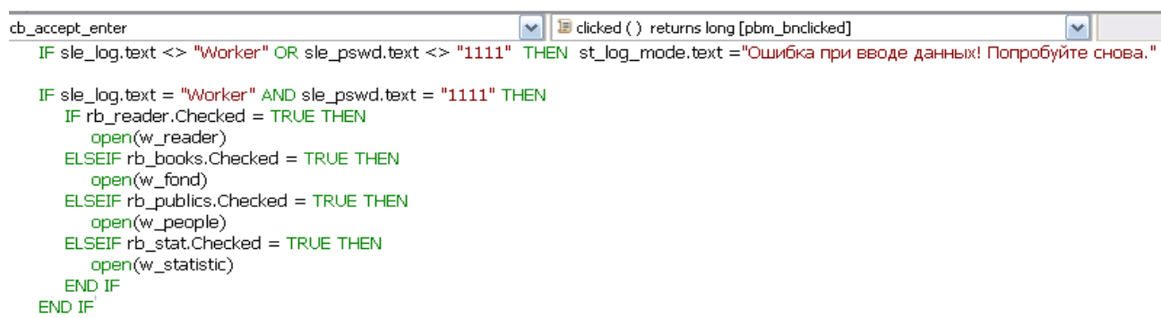
Рисунок 5. Обработчик события clicked кнопки «Подтвердить»
