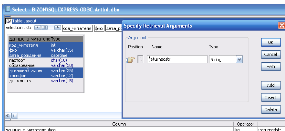
Рисунок 10. Настройка возвращаемых значений
