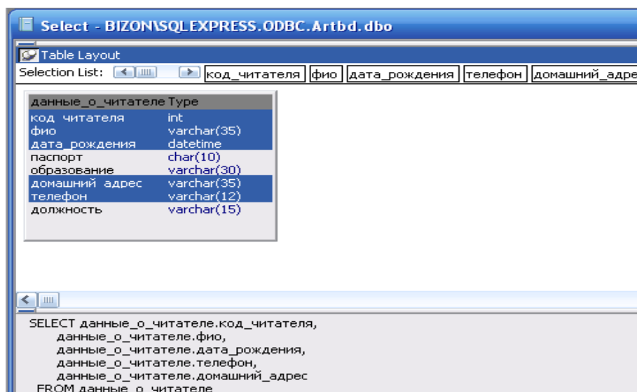
Рисунок 8. Создание SQL-запроса в PowerBuilder
