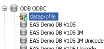
Рисунок 2. Подключенный профиль
