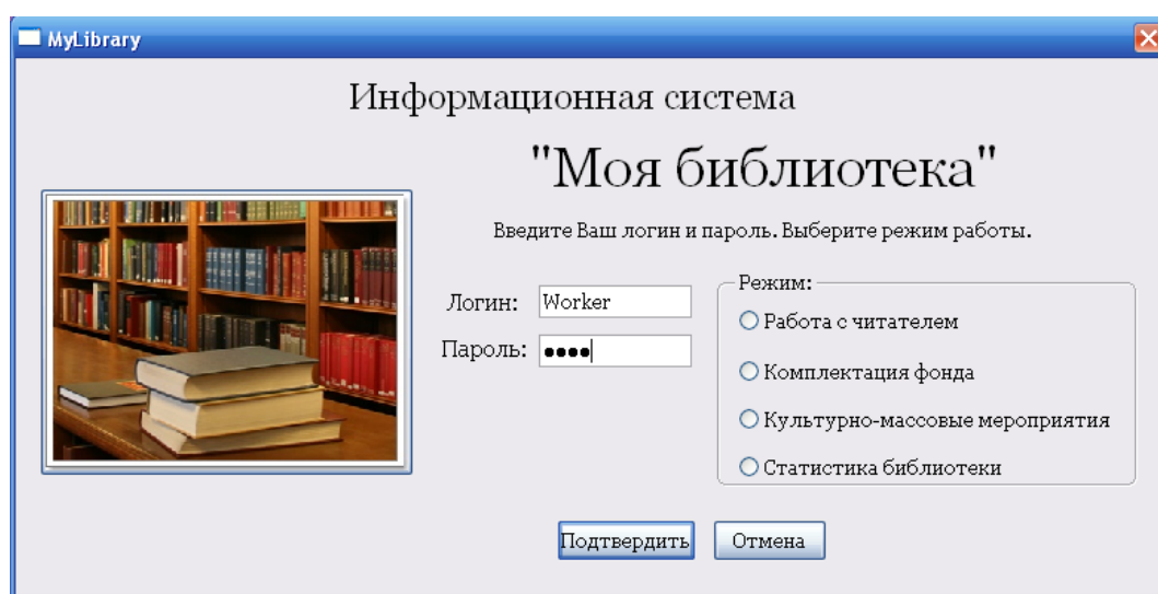
Рисунок 3. Окно авторизации
