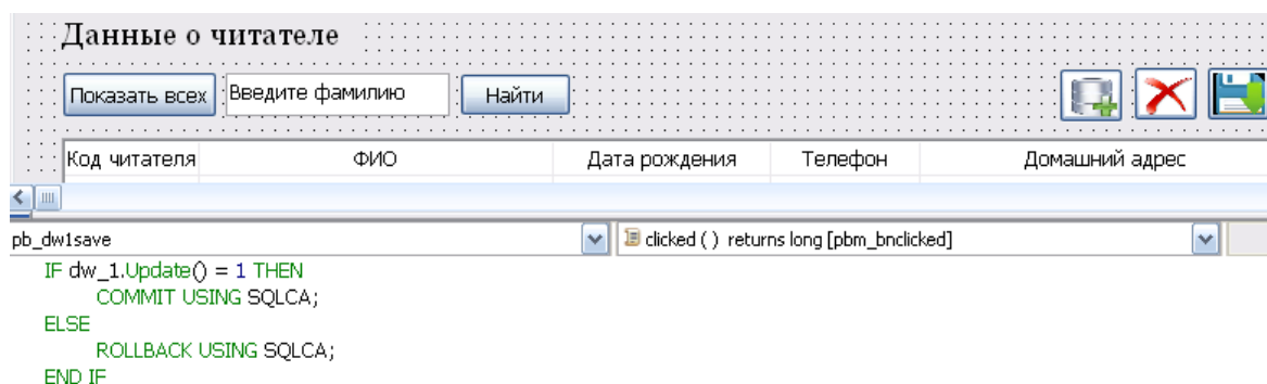
Рисунок 14. Скрипт кнопки-пиктограммы «Сохранить»
