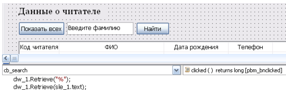
Рисунок 13. Скрипт для кнопки «Найти»
