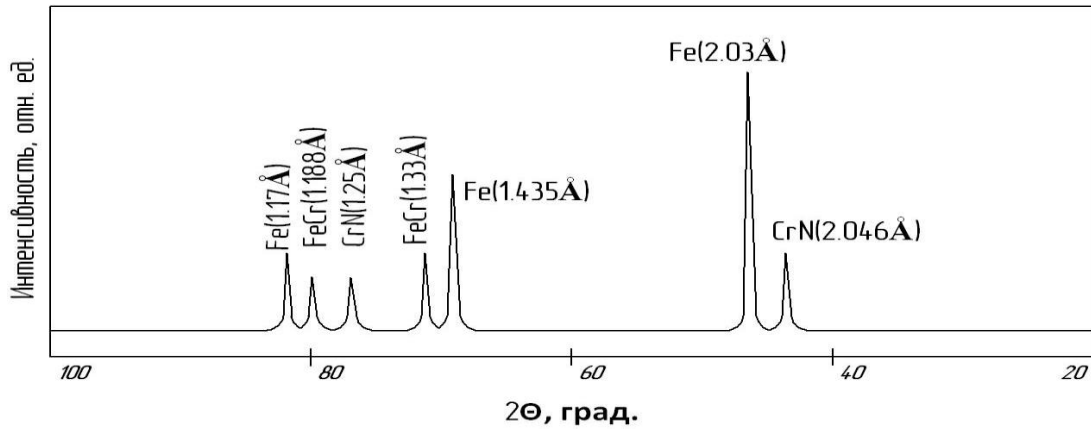
Рис. 2. Дифрактограмма покрытия, полученного на подложке СЧ 21 методом ионной имплантации при модификации поверхности ионами Cr и N (70мин).
