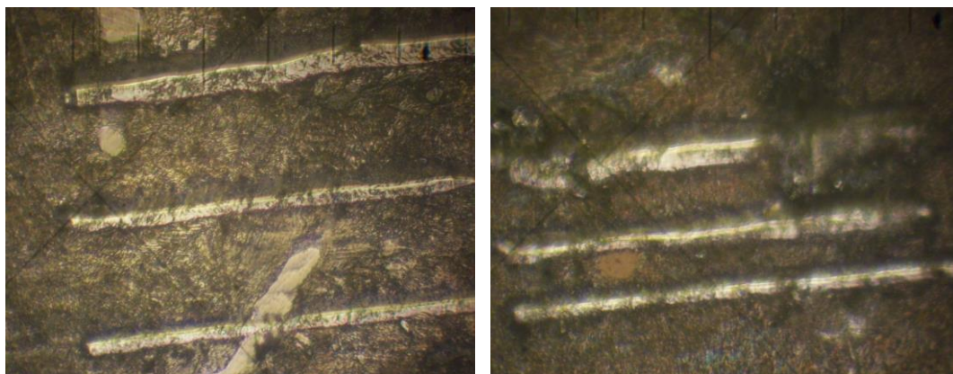
Рис. 5. Результаты царапания поверхности нитрида хрома на подложках серого чугуна СЧ 21 при нагрузке на индентор 15, 25, 35 г, а) время имплантации 10 мин, б) время имплантации 80 мин.
