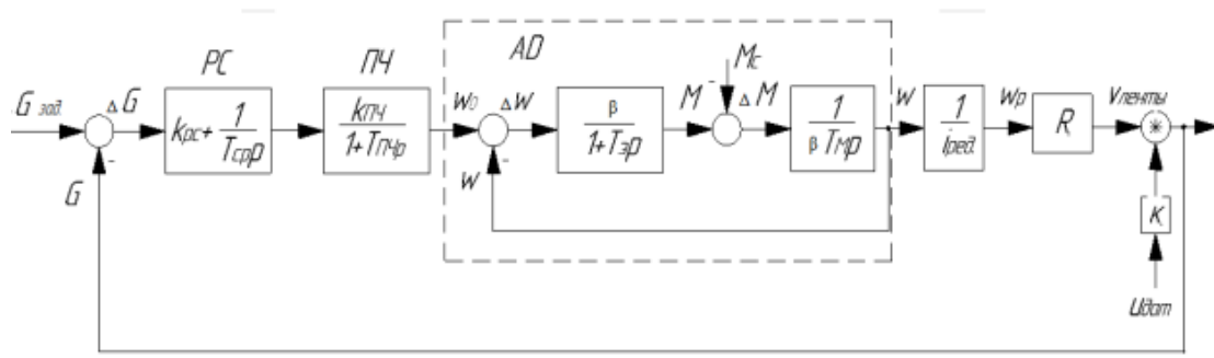
Рисунок 2 - Структурная схема системы управления: G_{зад} - заданная производительность, K_{рс} - пропорциональная составляющая регулятора, T_{срр} - интегральная составляющая регулятора, K_{ПЧ} - передаточный коэффициент преобразователя частоты, T_{ПЧр} - постоянная времени цепи управления преобразователя частоты, w - угловая скорость, \beta - модуль жесткости, T_{эр} - электромагнитная постоянная времени, T_{м} - электромеханическая постоянная времени, i_{ред} - передаточное число редуктора, R - радиус роликов, K - вес материала с датчика
