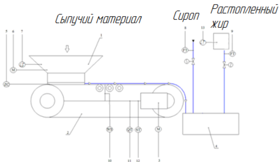
Рисунок 1 - Технологическая схема дозатора: 1-приемный бункер; 2- ленточный конвейер (дозатор); 3-мотор-редуктор с асинхронным двигателем для вращения ролика ленты; 4 — приемный бункер машины; 5- концевые выключатели для контроля схода ленты (справа и слева); 6- вибрационный привод бункера; 7- датчик уровня материала; 8 — датчик расхода сиропа; 9 — датчик расхода растопленный жир; 10 — датчик веса; 11 — датчик оборотов ленты; 12 — датчик скорости вала (энкодер); 13- ультразвуковой датчик уровня растопленного жира.
