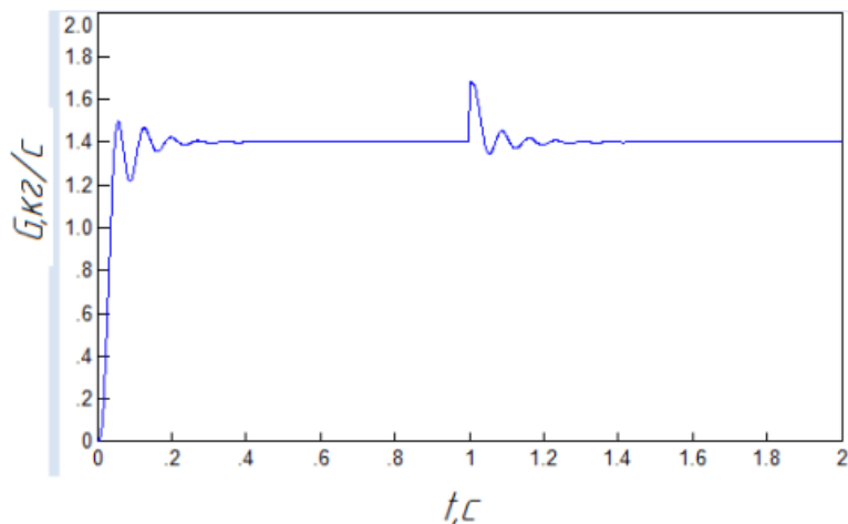
Рисунок 3 - График системы управления технологическим процессом
