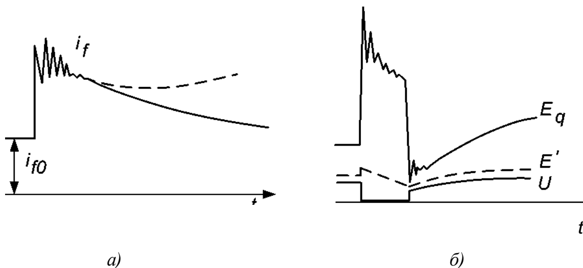
Рис. 3. Трехфазное КЗ вблизи шин генератора
