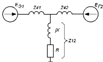
Рис.2. Преобразованная схема замещения.
