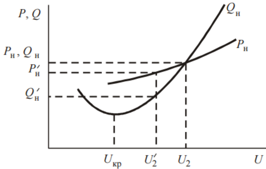
Рис. 1 – Статичні характеристики комплексного навантаження по напрузі
