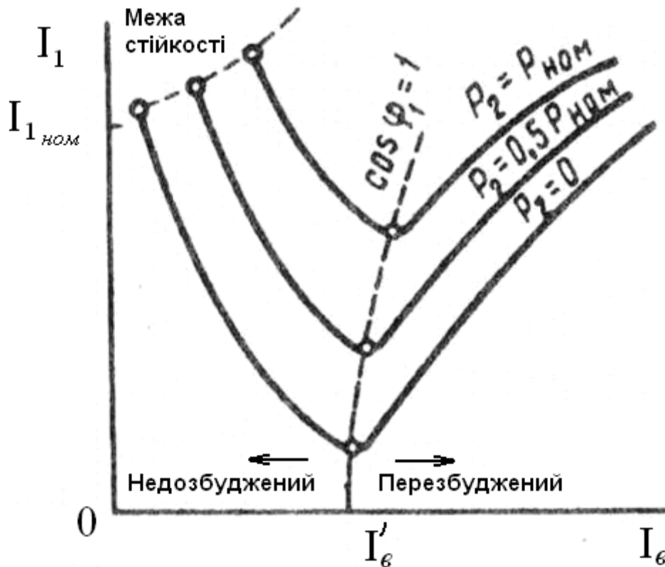
Рис. 4 – U-подібні характеристики синхронного двигуна
