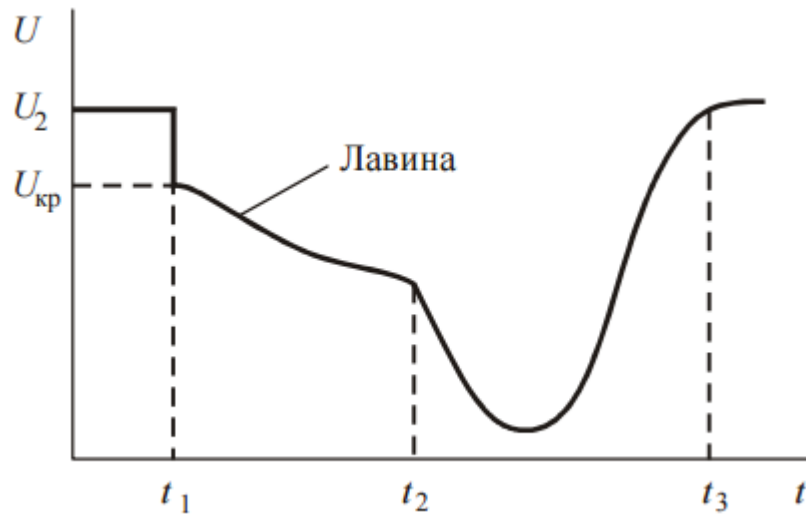
Рис. 2 – Розвиток лавини напруги
