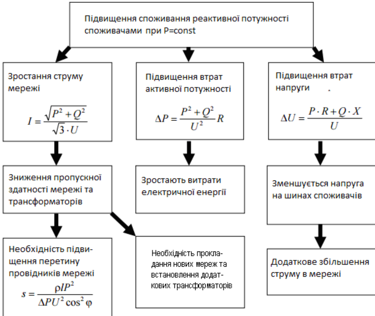
Рис. 3 – Проблеми в наслідок підвищення споживання реактивної потужності
