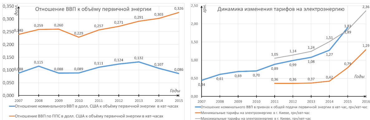
Рис. 5. Динамика отношения ВВП Украины к объёму первичной энергии
