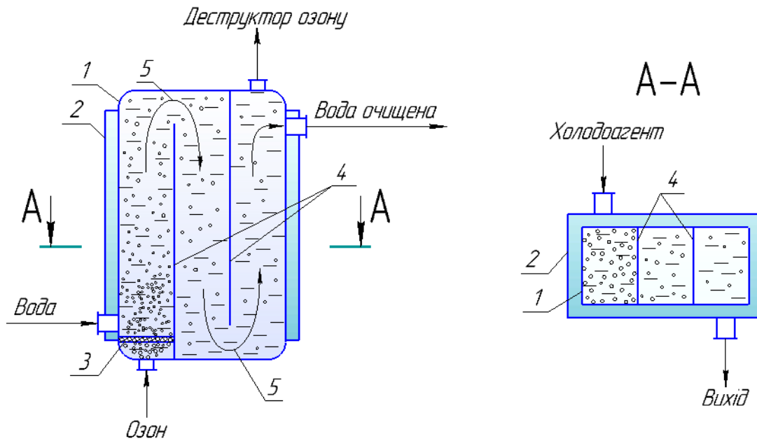
Рисунок 1. Схема озонатора
