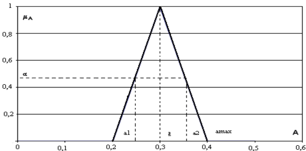
Рис. 1. – Функция принадлежности треугольного нечеткого числа A (составлено авторами на основе [1]).
