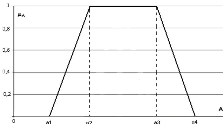
Рис. 2. – Трапецевидное нечеткое число (составлено авторами на основе [1]).
