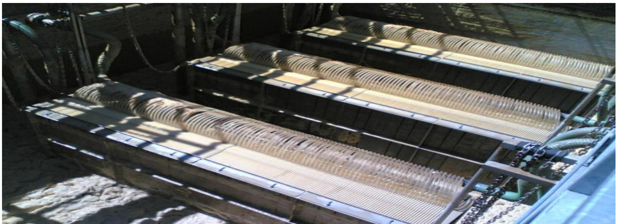
Рис. 3. Ультрафільтраційний мембранний модуль
