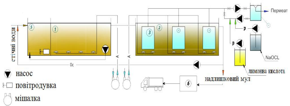
Рис. 2. Схема очищення стічних вод за допомогою мембранного біореактора: 1 – аеротенк; 2 – мембранний біореактор; 3 – мембранна біокасета; 4 – резервуар чистої води; 5 – денітрифікатор; 6 – станція зневоднення осаду; А – повітропровід; Р – трубопровід подачі реагенту; Ос – трубопровід циркулюючого мулу; Об – відвід зневодненого осаду.
