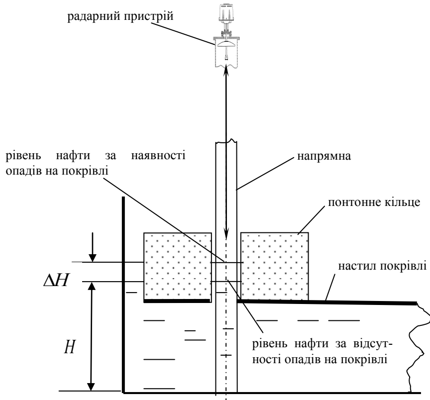
Рис. 2 Схема затвору плаваючої покрівлі (ущільнення умовно не показані) (складено автором на підставі [3, с. 147])
