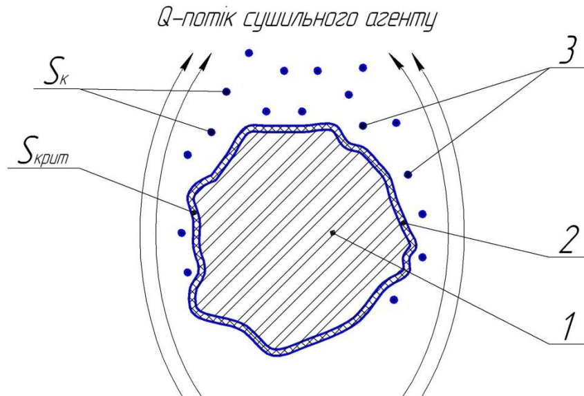
Рисунок 1 – Частинка пасти діоксиду титану в потоці теплоносія
