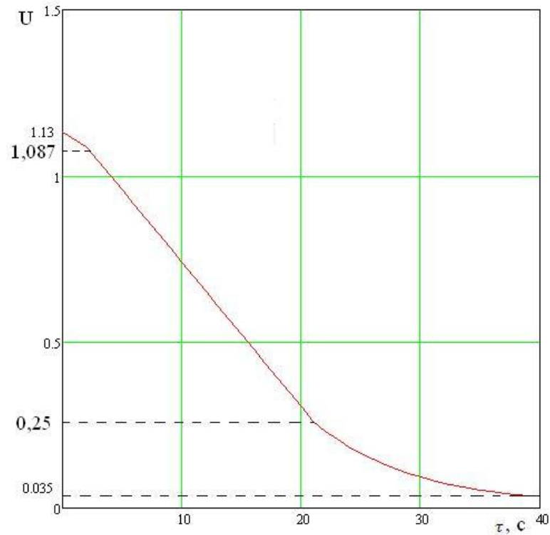
Рисунок 2 – Залежність вологовмісту частинки діоксиду титану від часу сушіння
