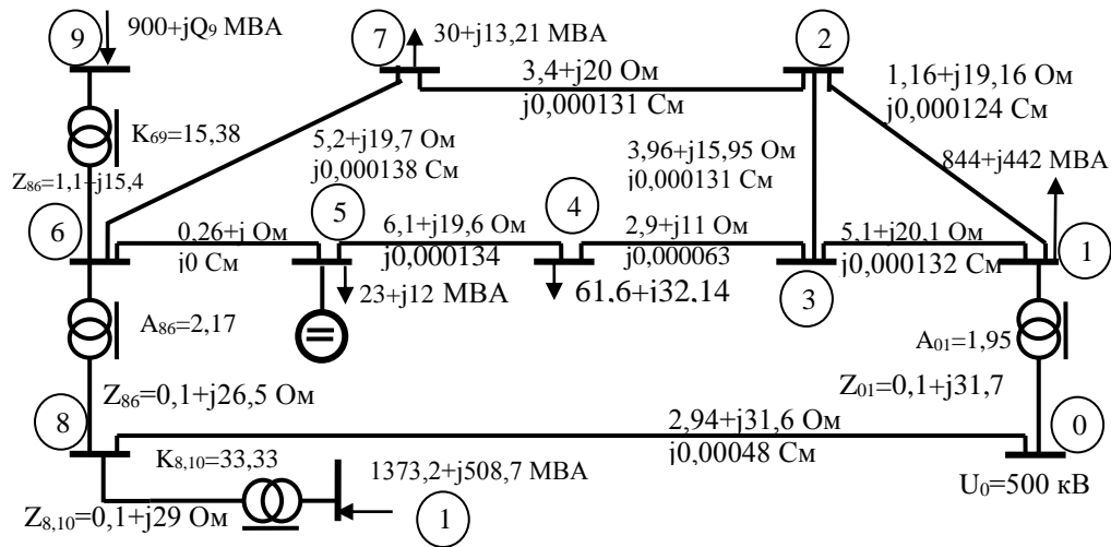
Рис.1. Схема электрической сети.
