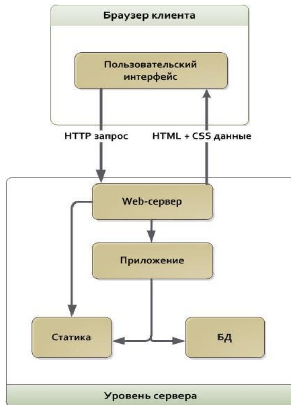
Рис. 1. Архитектура web -приложения
